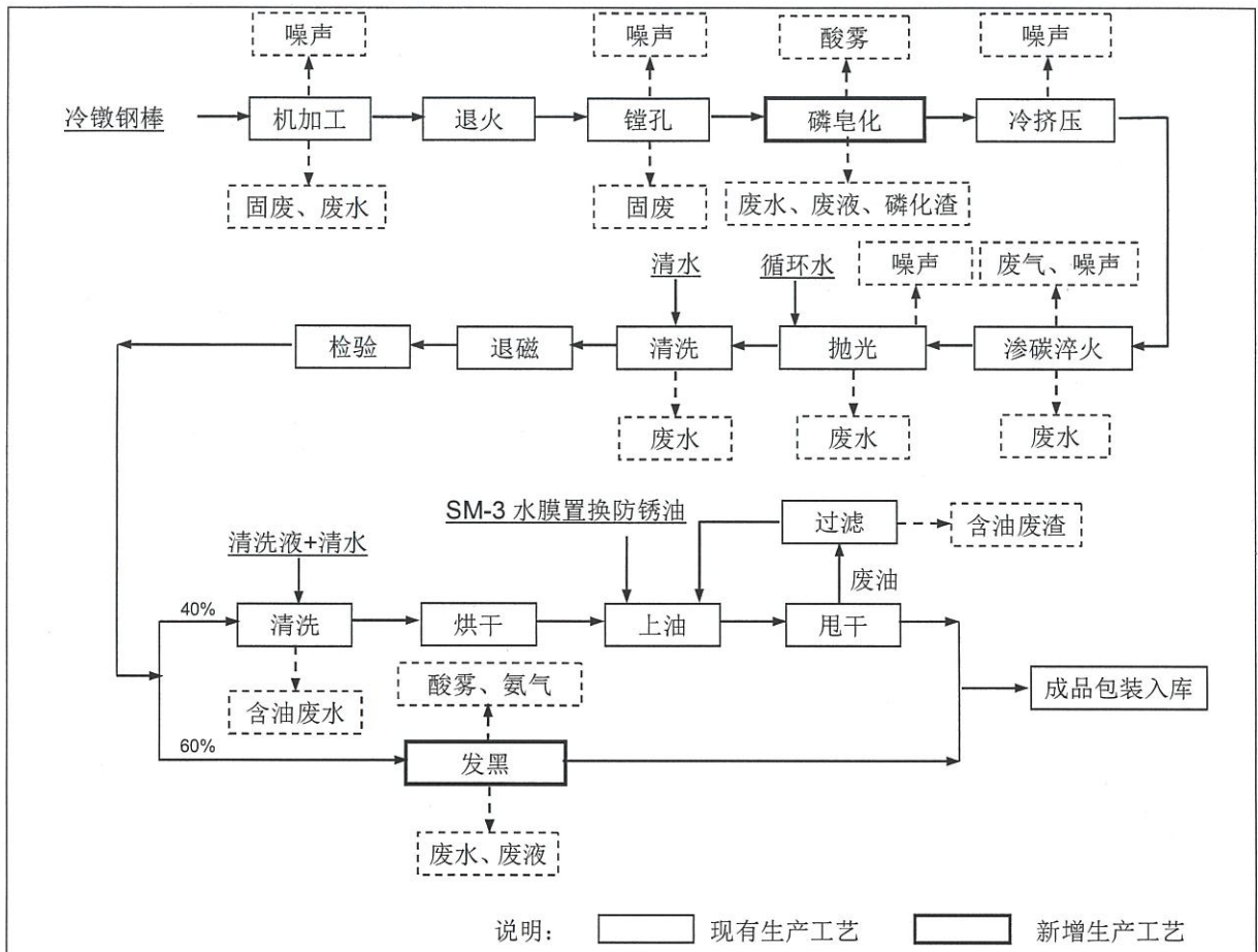
图 1 气门弹簧座生产工艺流程图
